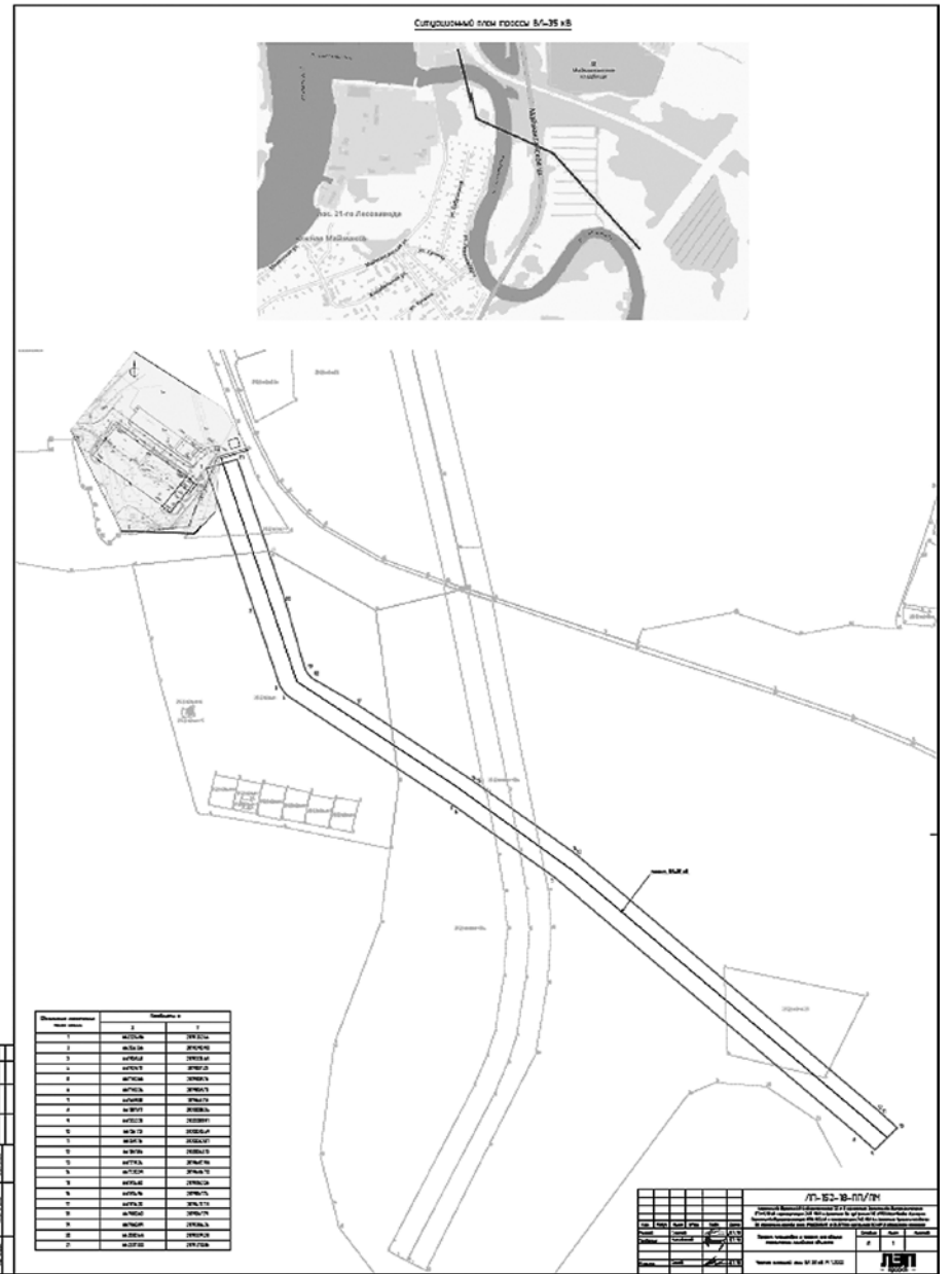
Приложение № 2 к проекту планировки территории линейного объекта «Участок двухцепной ВЛ-35 кВ протяженностью 1,25 км в г.Архангельске Архангельской области»
